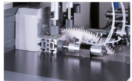
Pilový automat SA 142/37
