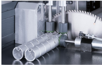
Pilový automat SA 142/37
