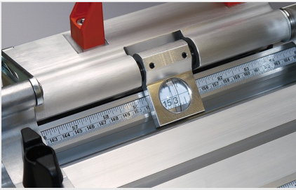
Dorazový a měřicí systém MMS 100
