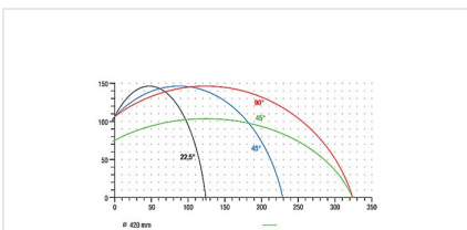
Pokosová pila MGS 105
