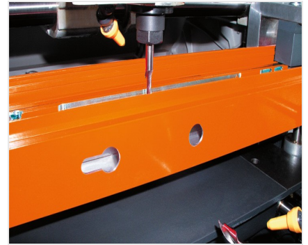
2vřetenová kopírovací fréza KF 78/23
