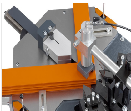
Lis pro spojování rohů EP 120
