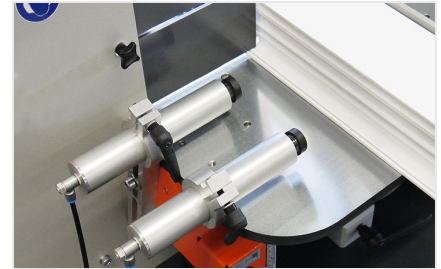
Čelní fréza AF 222/02
